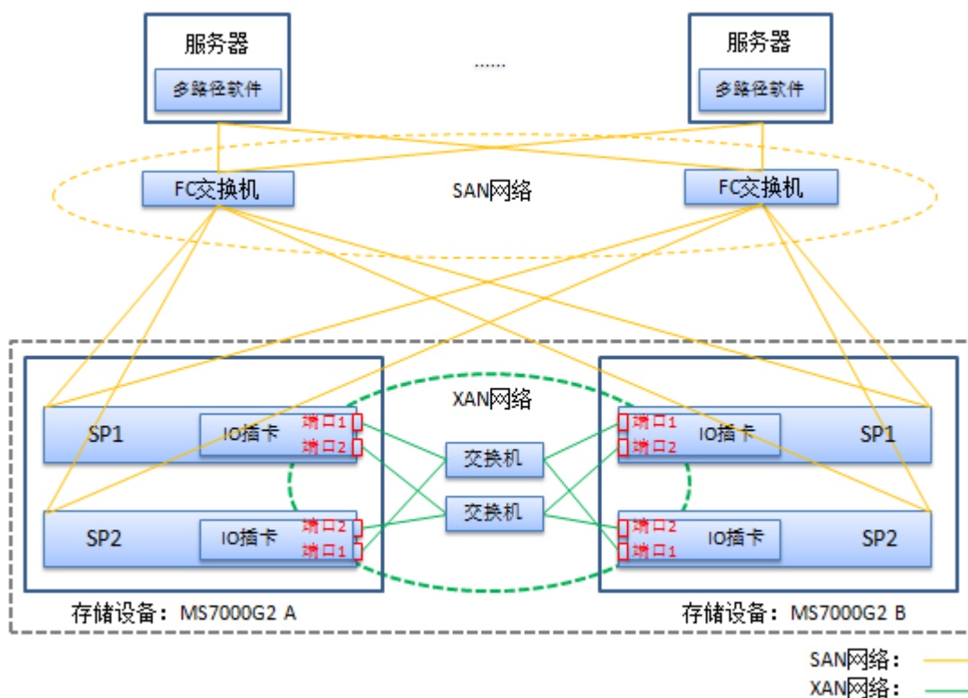
图4-2 双控 XAN 典型组网图（交换机连接）
