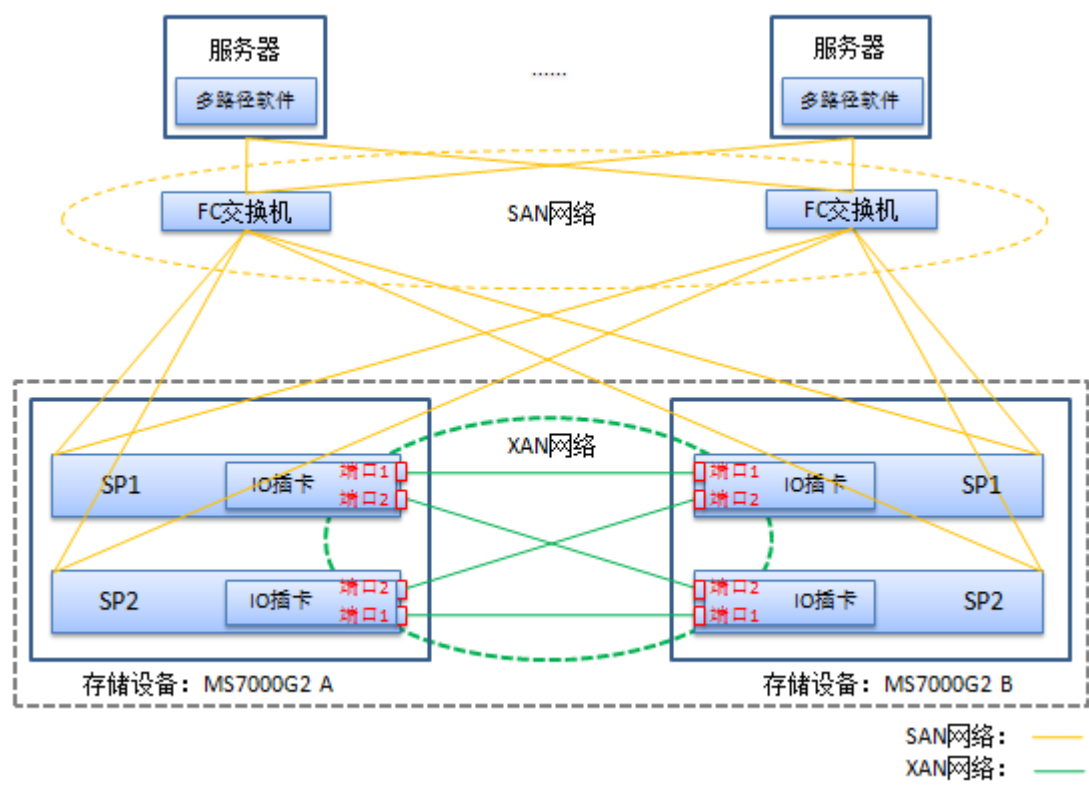
图4-1 双控 XAN 典型组网图（MESH 直连）
