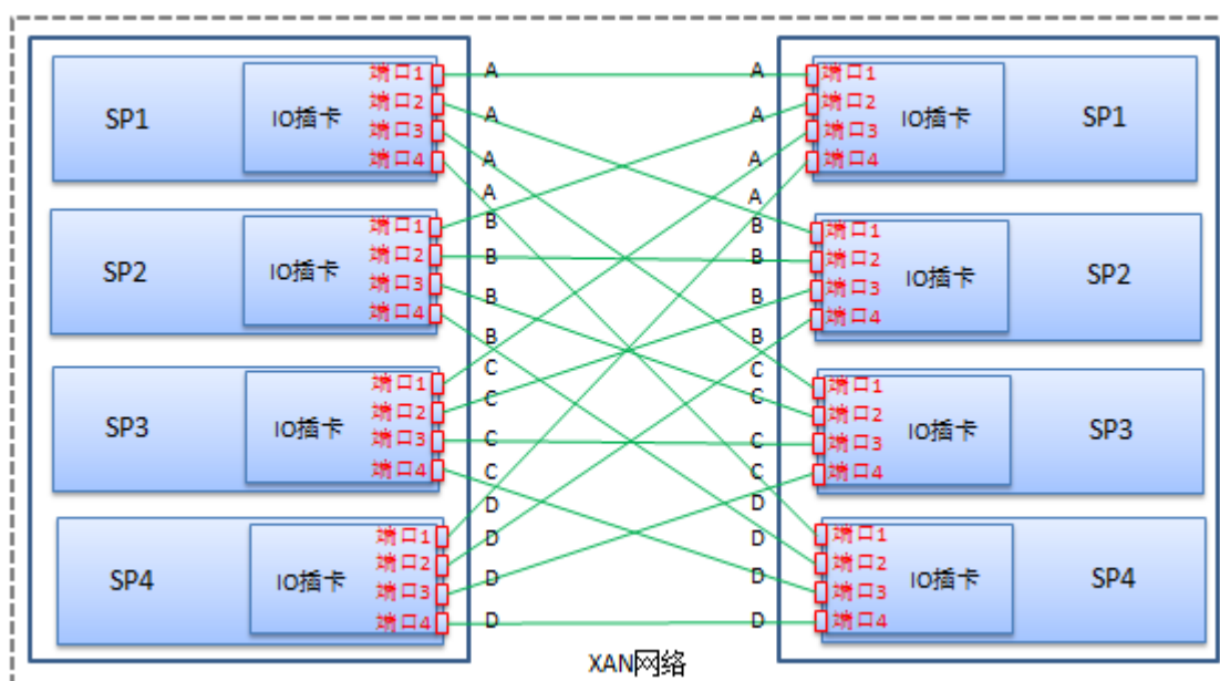
图4-6 四控 XAN 网络（MESH 直连）链路编号示意图
