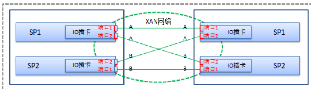
图4-5 双控 XAN 网络（MESH 直连）链路编号示意图
